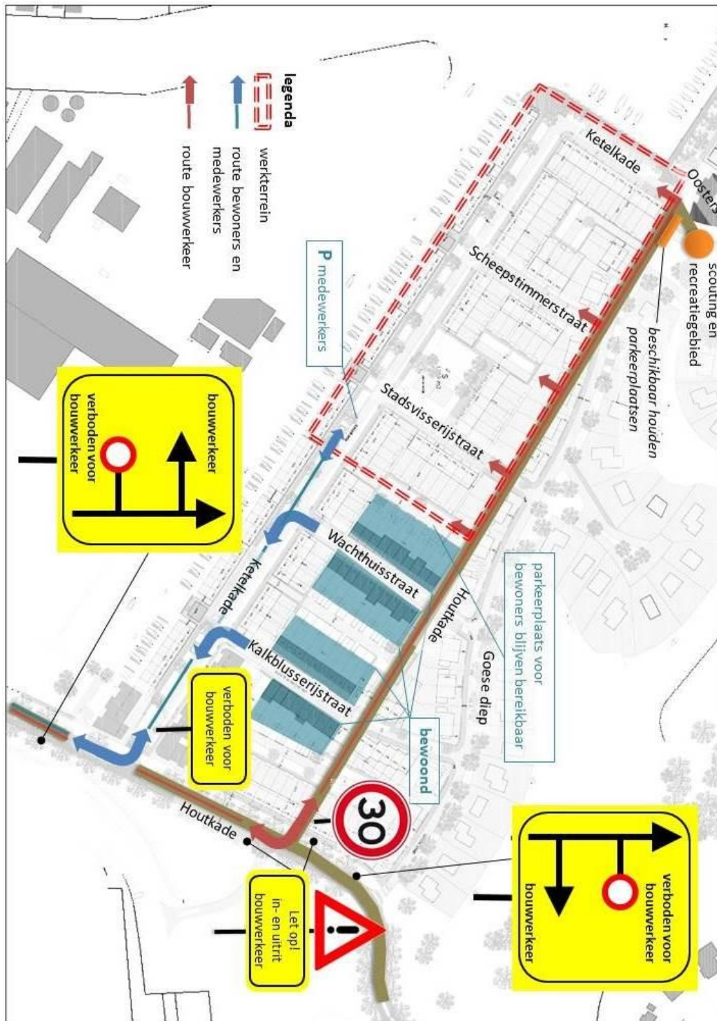
Figuur 1 Bereikbaarheid | verkeersstromen bouwplaats Goese Diep
